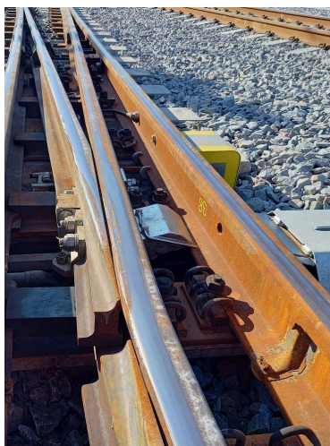
obrázek 69 – PHS přiléhající ke kolenové kolejnici (křížovatková výhybka)
