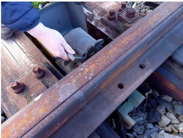
obrázek 129 – Stav po sklopení ochranné skříňky výměnového zámku (uchopení rukojeti zámku)
