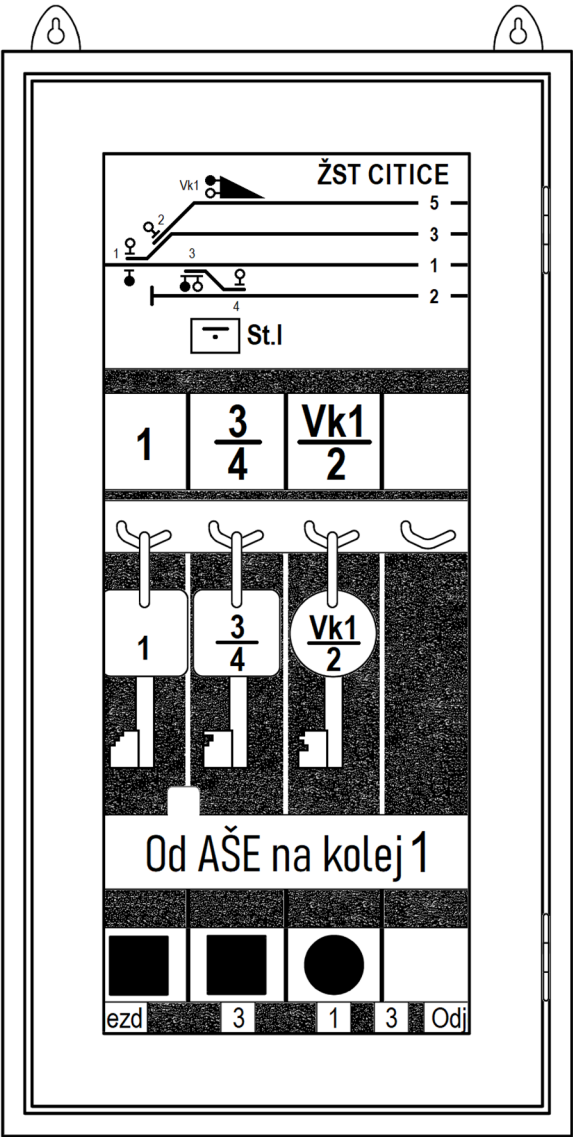
obrázek A.45 – Tabule k zavěšování hlavních klíčů v uzamykatelné skřínce
