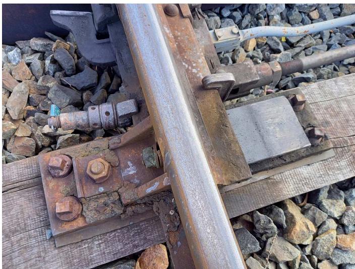
obrázek 141 – Příklad uzamknutí výhybky při osazení přenosného výměnového zámku v prvním mezipražcovém poli
