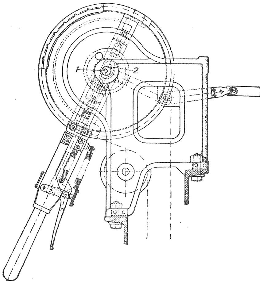
obrázek A.26 – Trojstavná páka
