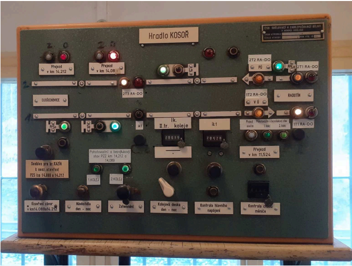
obrázek 383 – Příklad doplněné indikační desky hradlového přístroje
