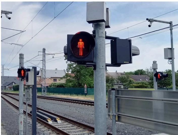
obrázek 415 – Světelný signál „Stůj“ dávaný zdrojem světelné signalizace (přerušované červené světlo)
