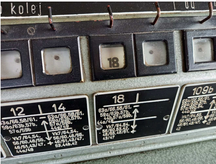
obrázek 286 – Číslo na kolejovém číselníku
