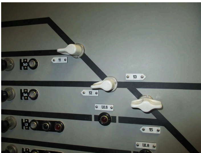
obrázek 272 – Výměnový řadič (dvoupolohový, umístěný v kolejovém plánu)
