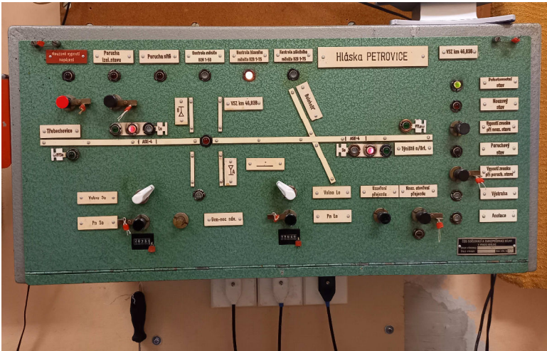
obrázek 379 – Příklad indikační desky s ovládacími a indikačními prvky na hlásce
