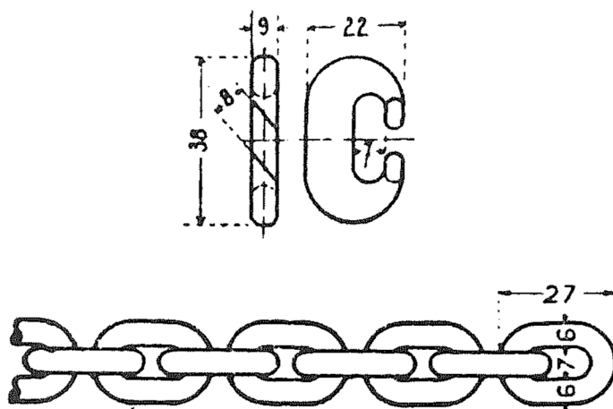
obrázek A.21 – Hradlový řetěz a spojovací článek
