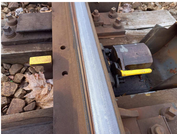
obrázek 103 – Výměnový zámek
