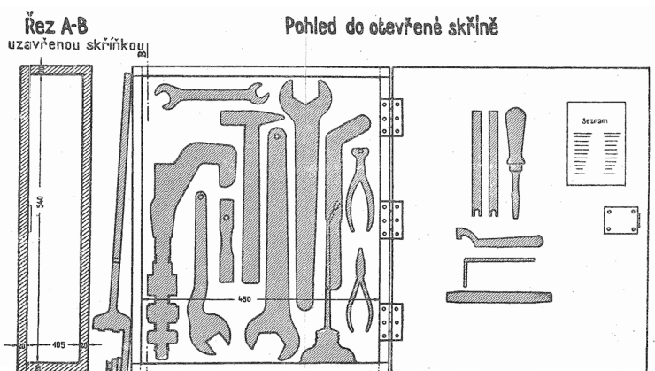
obrázek A.48 – Příklad skříně s náradím
