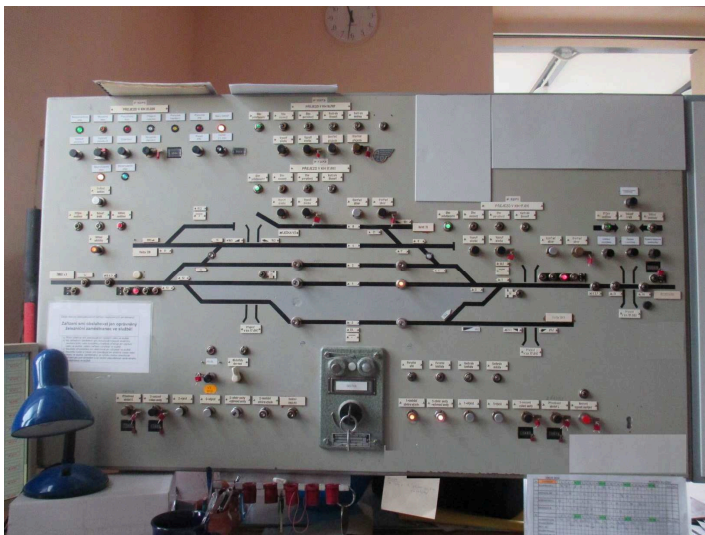
obrázek 360 – Řídící stavědlo SZZ TEST s řídicím stavědlem a závislými výhybkářskými stanovišti
