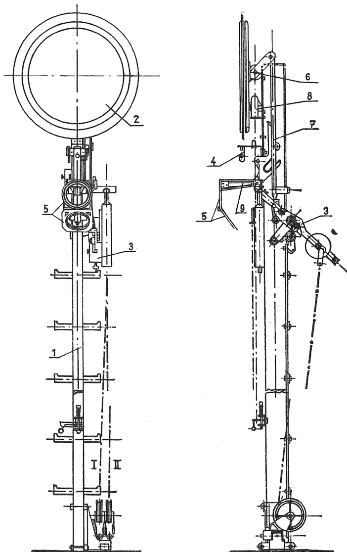
obrázek A.18 – Samostatná předvěst (mechanická)
