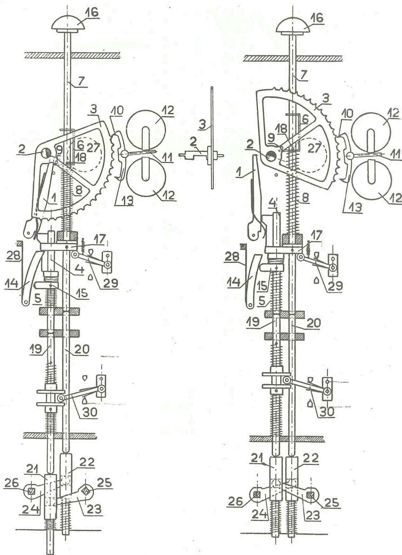
obrázek A.35 – Hradlový závěr na střídavý proud
