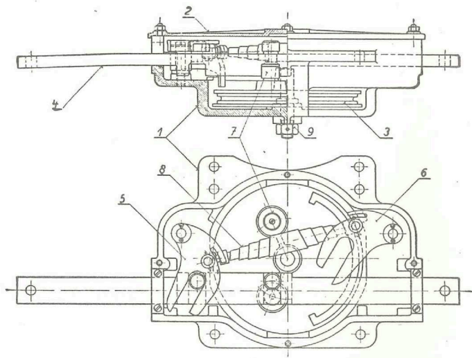
obrázek A.5 – Přestavník s pružinou
