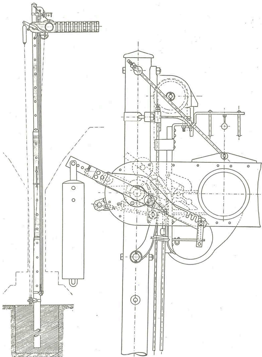
obrázek A.13 – Jednoramenné mechanické návěstidlo
