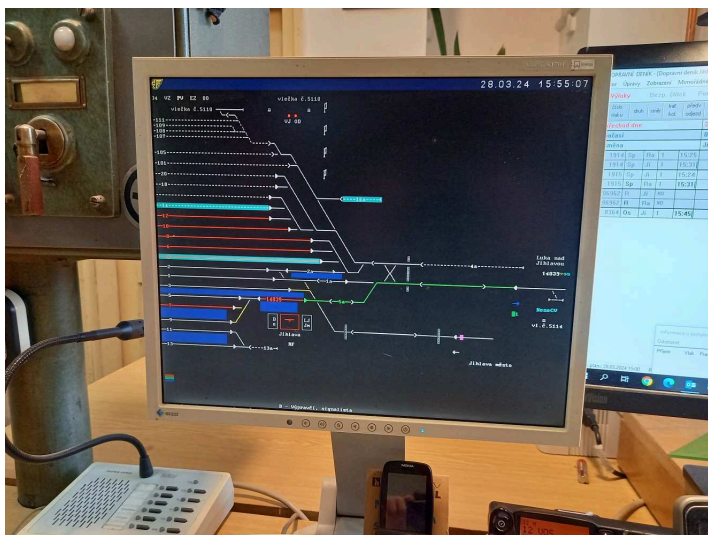
obrázek 371 – Terminál pro zadávání čísel vlaků (zobrazení reliéfu kolejíště sousední dopravy)
