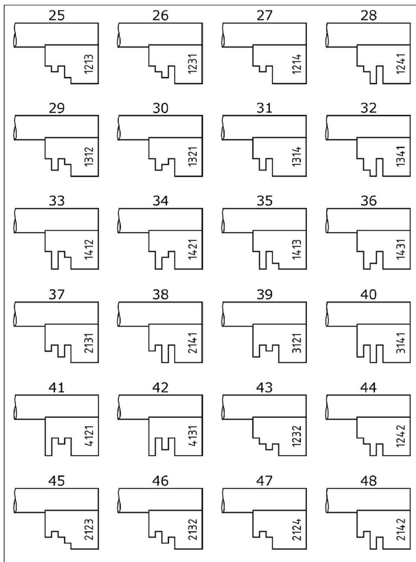
obrázek A.44 – Typy klíčů mechanických zámků (pokračování)
