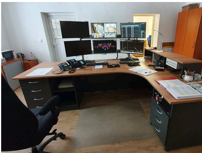
obrázek 372 – Jednotné obslužné pracoviště SZZ K-2002
