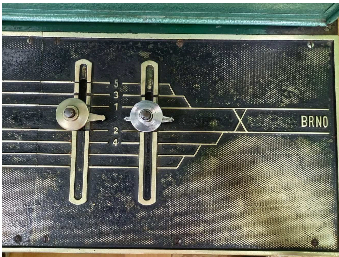
obrázek 288 – Detail kolejového plánu (kolejový reliéf) na horní desce závěrové skříně řídicího přístroje
