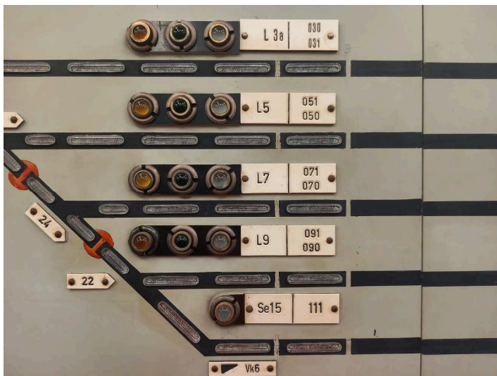
obrázek 346 – Detail indikační desky RZZ cestového systému se skupinově přestavovanými výchlejkami (výkolejkami) s číslicovou volbou
