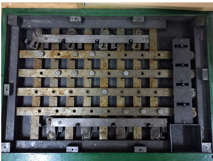
obrázek 248 – Detail pravítek ústředního zámku (bez čelního krytu)
