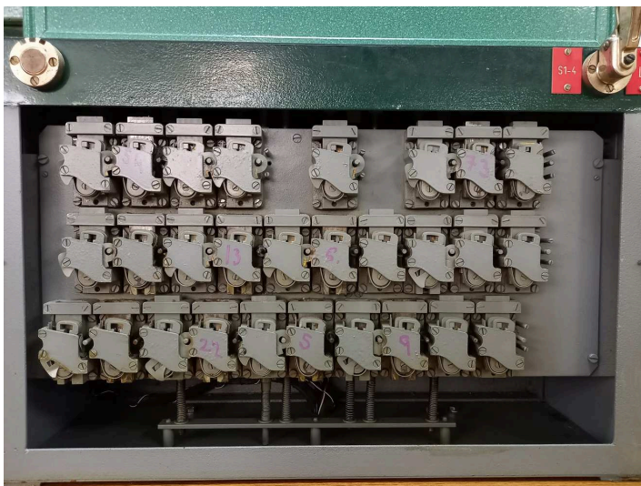
obrázek 250 – Detail klíčového (bubnového) přístroje (bez čelního krytu)
