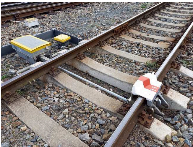
obrázek 85 – Výkolejka pravá (novější typ)
