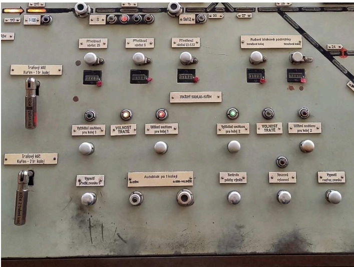
obrázek 389 – Ovládací a indikační prvky automatického bloku
