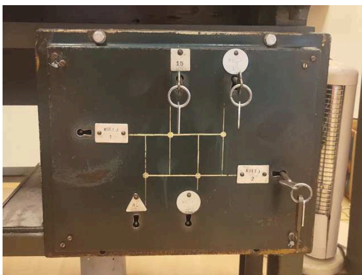
obrázek 246 – Ústřední zámek (potřebné tvary štítků vyznačeny u klíčových otvorů)
