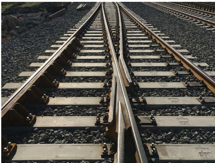
obrázek 74 – Srdcovka s průběžnou kolejnicí
