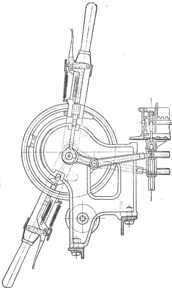
obrázek A.27 – Dvojitá páka
