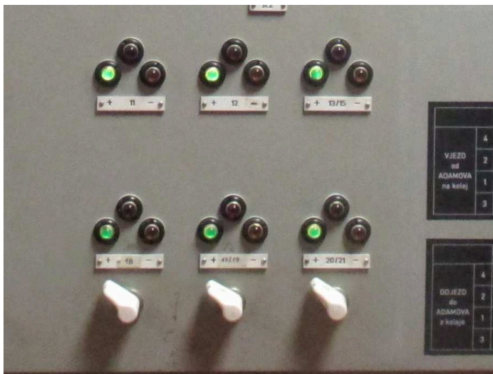
obrázek 273 – Výměnový řadič (dvoupolohový, umístěný mimo kolejový plán)
