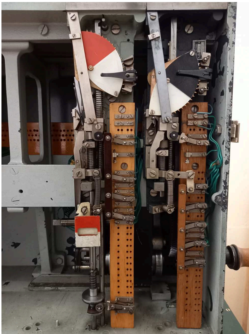
obrázek 296 – Hradlové závěry a náhradní západka (sejmutý kryt skříně)
