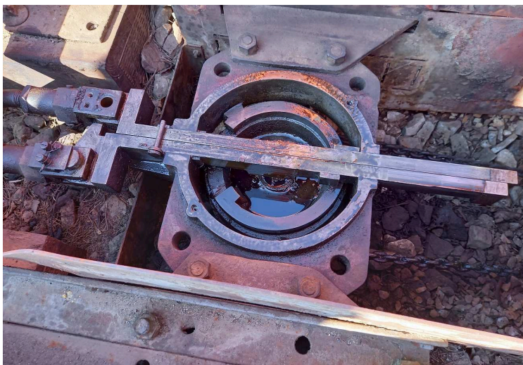
obrázek 183 – Sejmутý kryt mechanického záporníku výhybky (foceno během vypnutí z ústředního závorování)
