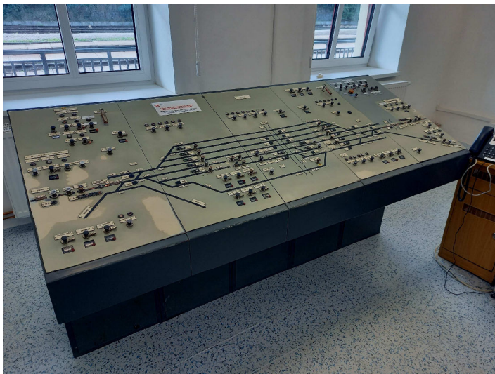
obrázek 362 – Řídící stavědlo SZZ TEST s řídícím stavědlem a závislými stavědly
