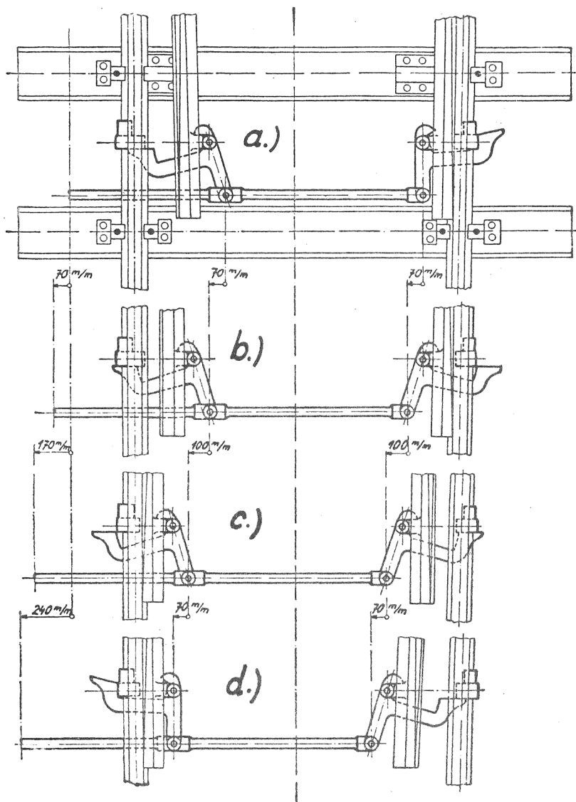
obrázek A.10 – Chod hákového závěru výhybky s vyznačením změn fází v provedení s postupným chodem jazyků
