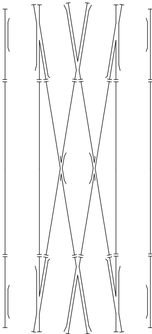
obrázek B.19 – Střed dvojité kolejové spojky (prodloužené křídlové kolejnice plnicí i funkci přídržnice)
