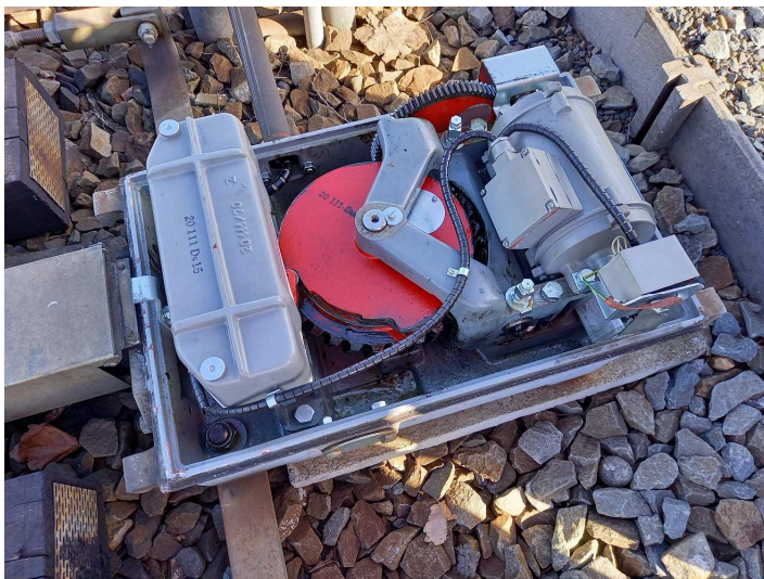
obrázek 176 – Detail elektrického přestavníku bez horního krytu
