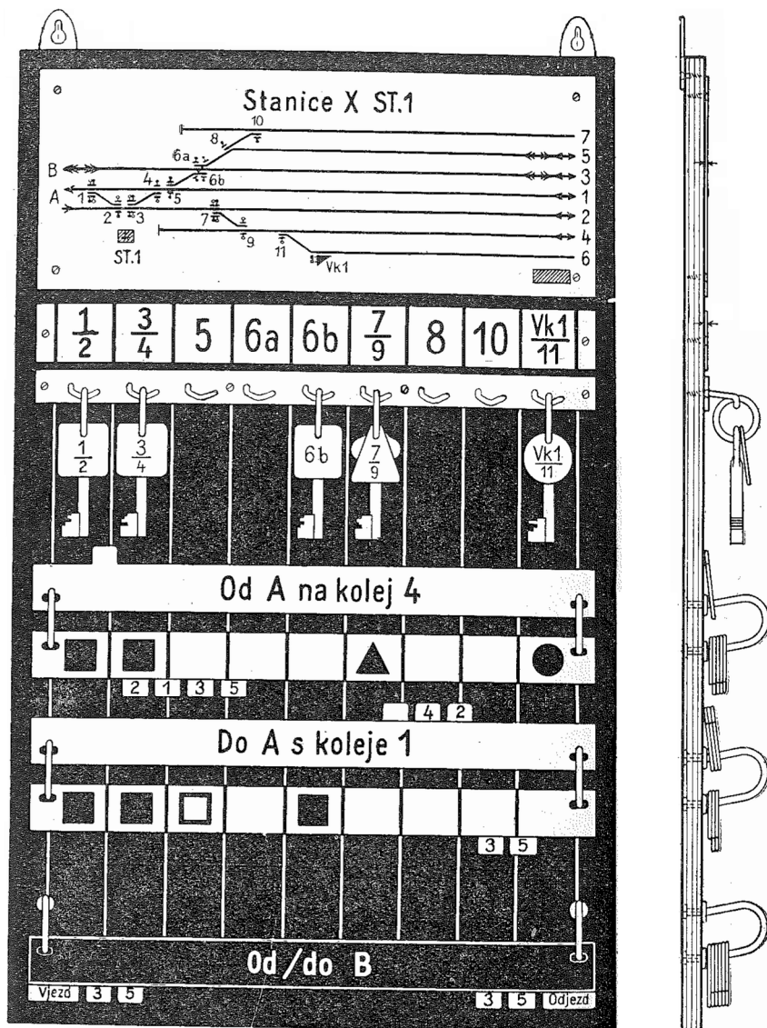
obrázek A.46 – Tabule k zavěšování hlavních klíčů
