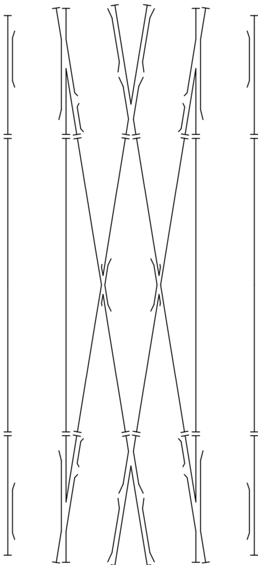
obrázek B.18 – Střed dvojité kolejové spojký (přidrznice oddělené od křídlových kolejnic)
