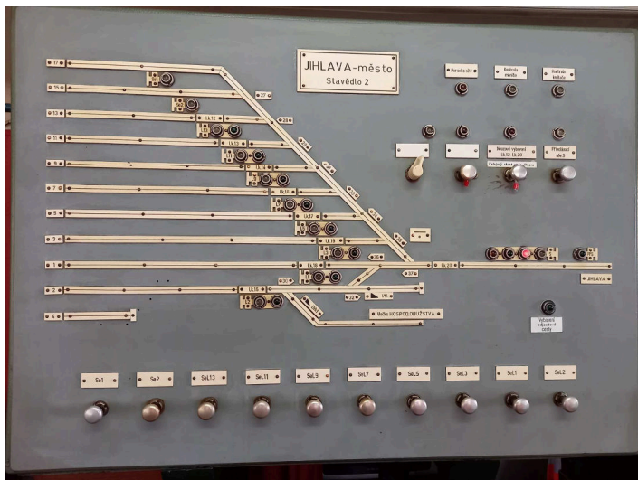
obrázek 28 – Příklad indikační desky (starší typ)
