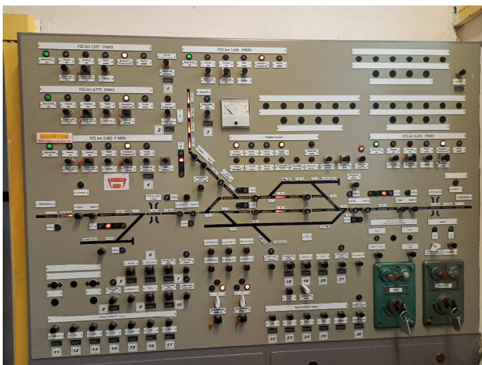
obrázek 356 – Ústřední stavědlo SZZ TEST s KÚ – indikační deska
