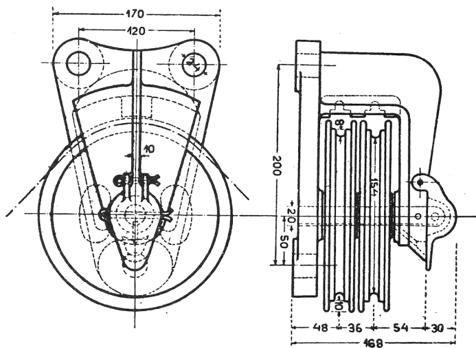
obrázek A.20 – Odbočná kladka
