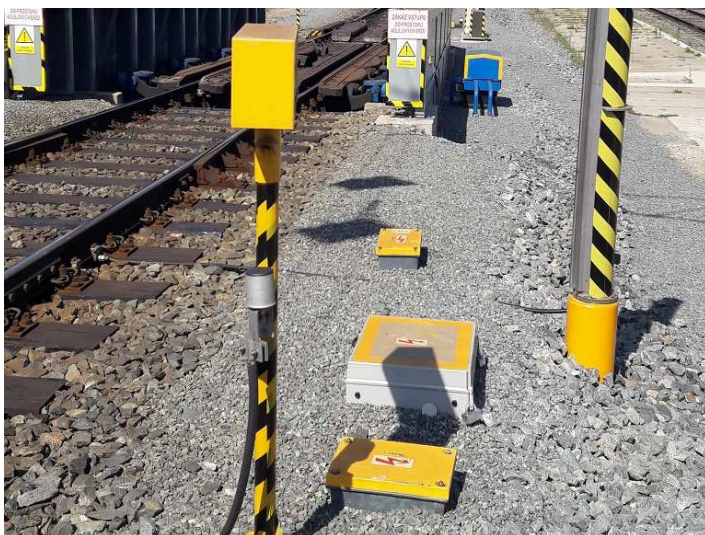
obrázek 440 – Optická závora za kolejovou brzdou (sloup vpravo)
