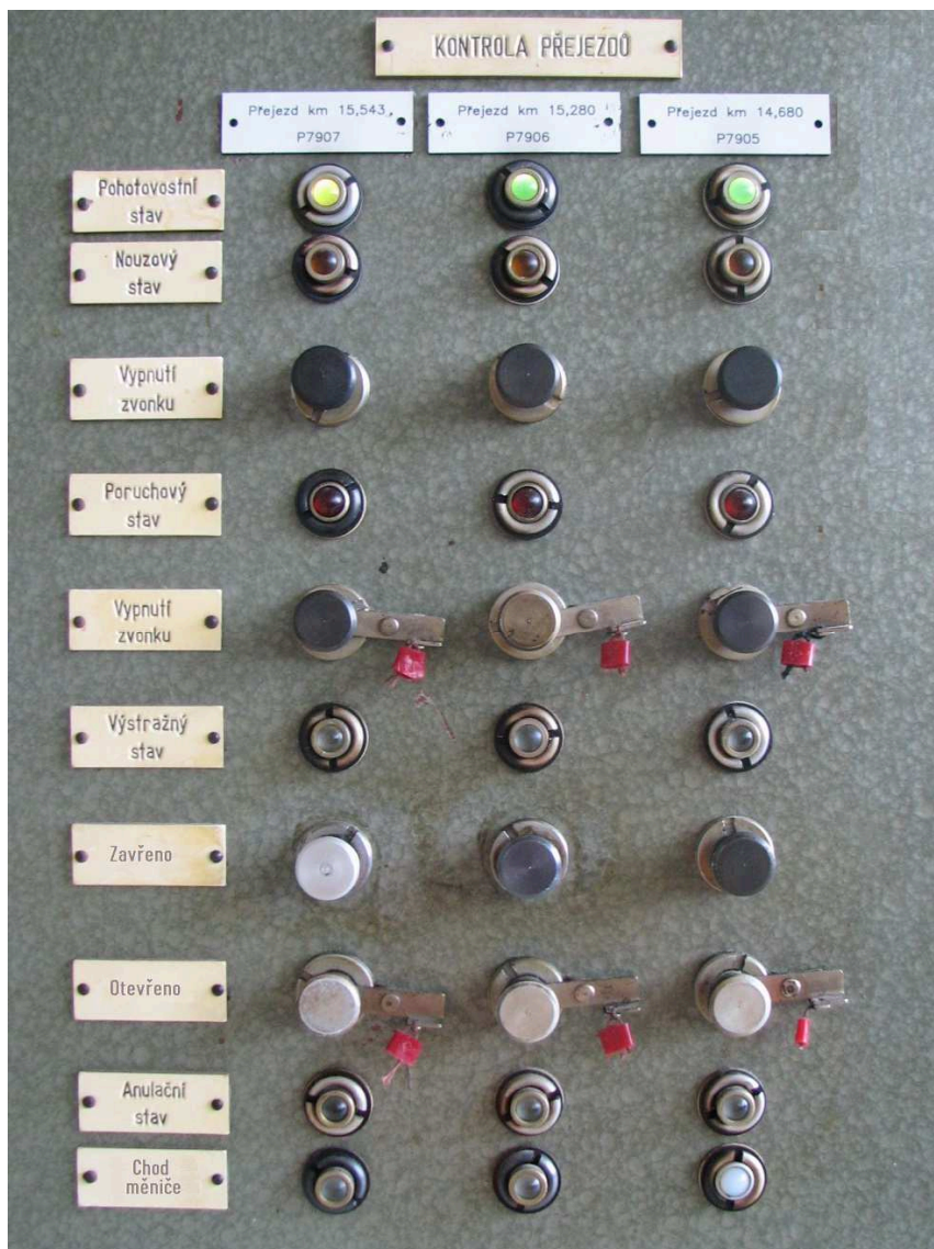
obrázek 411 – Ovládací skříňka PZS typu AŽD 71
