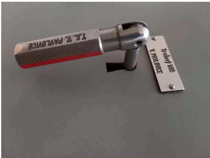
obrázek 24 – Traťový klíč (uzamknutý v elektrickém zámku)
