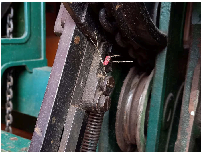
obrázek 268 – Úsmyčný kolíček na rozřezné stavěcí páce, s plombou na drátu
