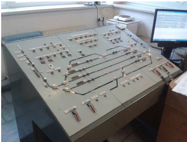
obrázek 336 – Ovládací stůl reléového ZZ (dále také „RZZ“) s jednotlivě přestavovanými výhybkami (výkolejkami)
