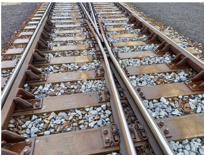
obrázek 71 – Srdcovka, včetně křídlových kolejnic
