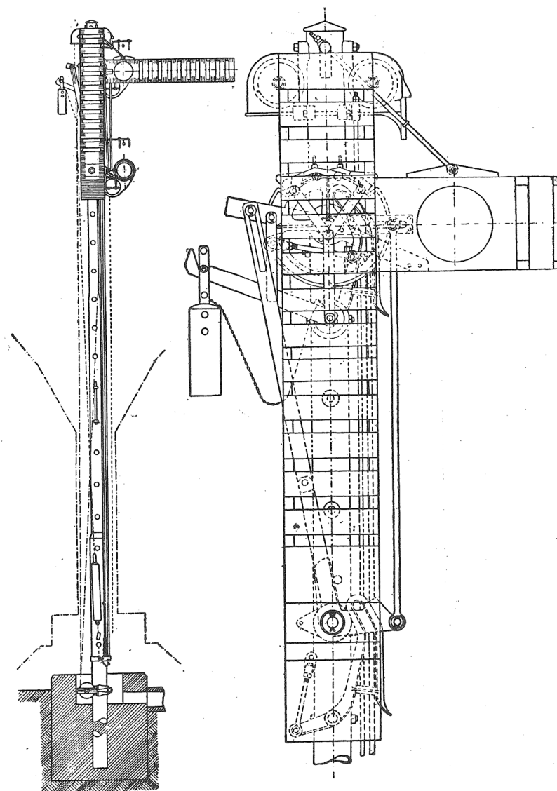
obrázek A.16 – Dvouramenné mechanické návěstidlo
