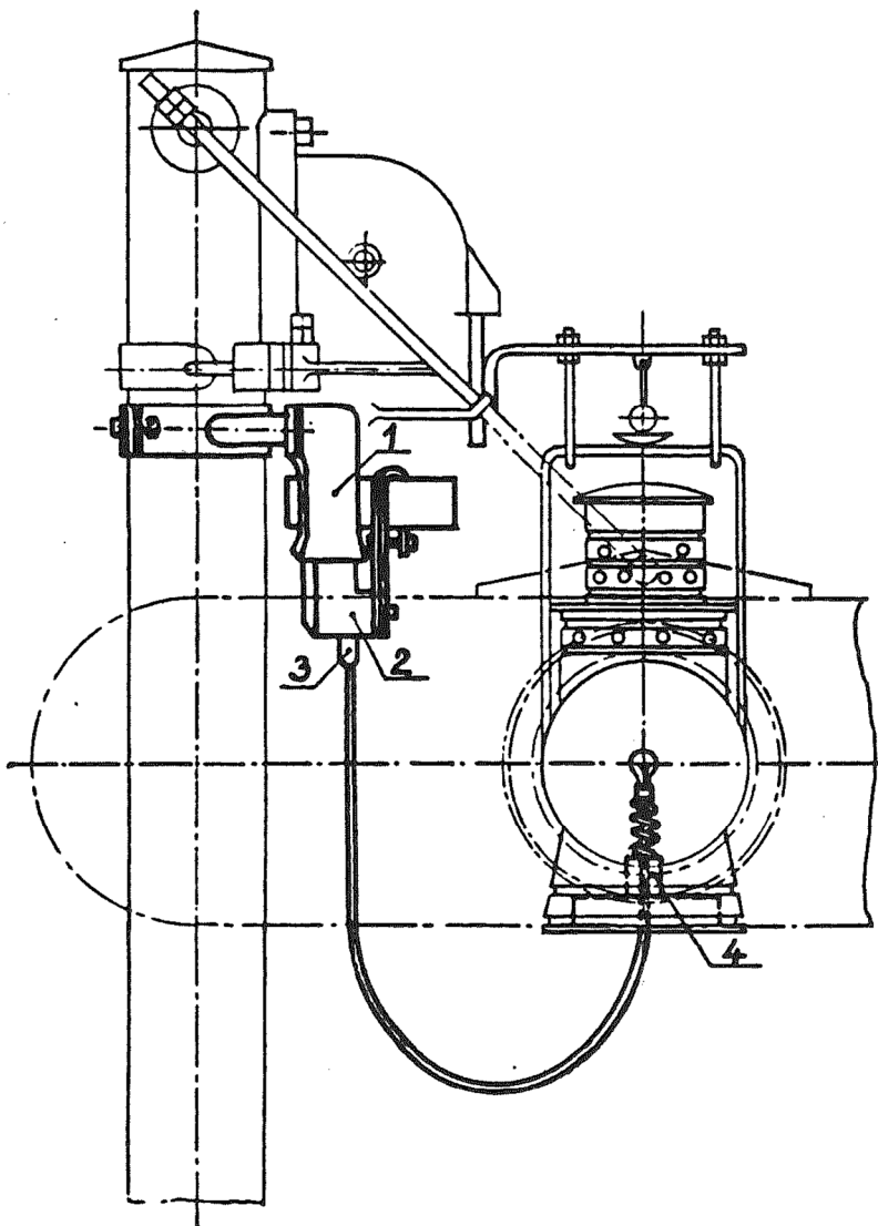
obrázek A.19 – Elektrické osvětlení mechanických návěstidel
