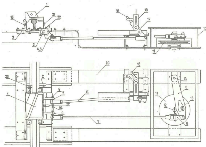
obrázek A.8 – Mechanický přestavník pro výkolejku
