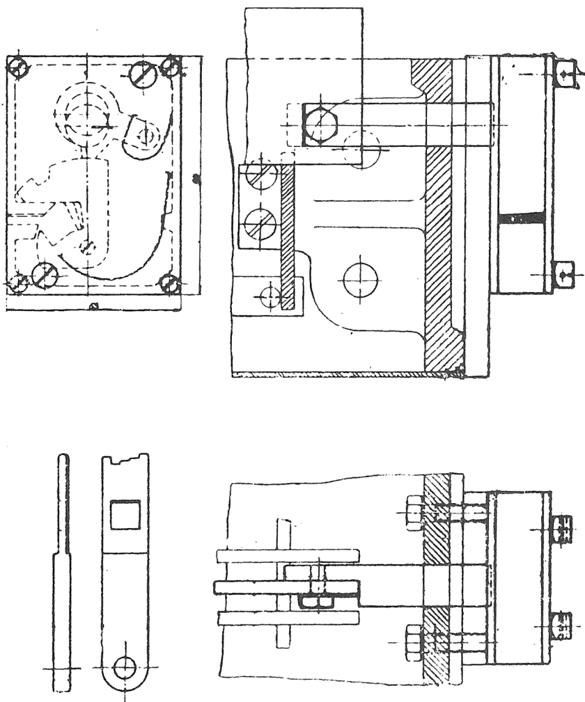
obrázek A.30 – Zástrčkový zámek a klíč zástrčkového zámku (vlevo dole)
