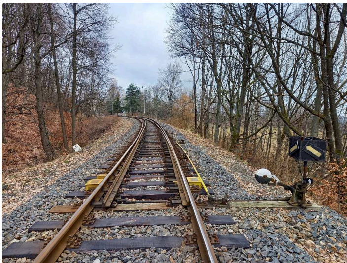
obrázek 50 – Jednoduchá výhybka oblouková jednostranná
