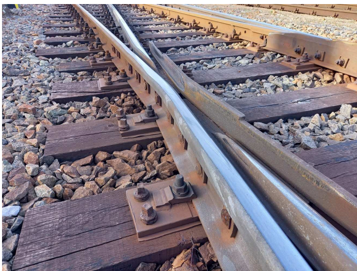
obrázek 75 – Kolenová kolejnice (součást dvojité srdcovky)
