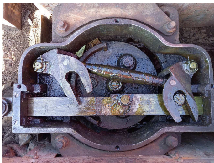
obrázek 159 – Vnitřní část mechanického přestavníku s pružinou (rozřezného) pro výhybku (sejmutý kryt)
