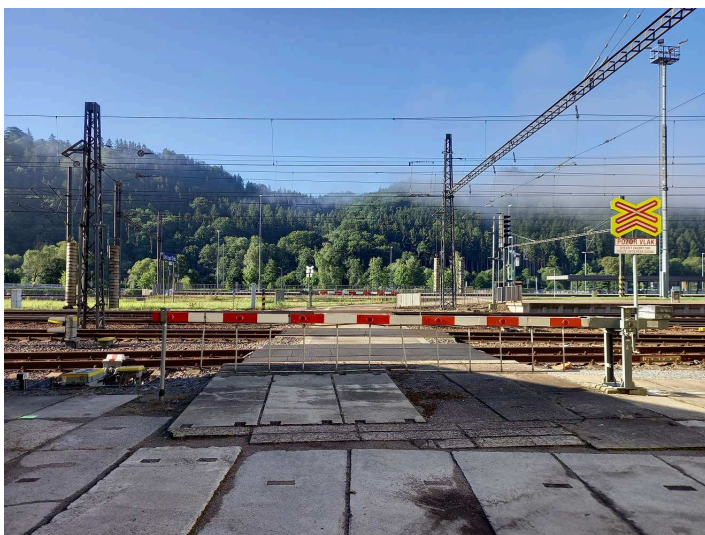
obrázek 404 – Přejezd s PZM 2U
