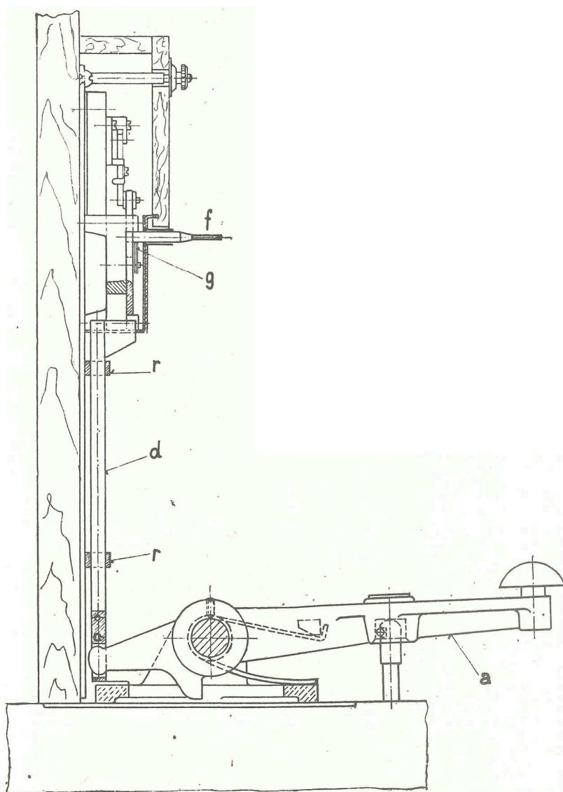
obrázek A.34 – Hradlové tlačítko s dotekovým klíčem
