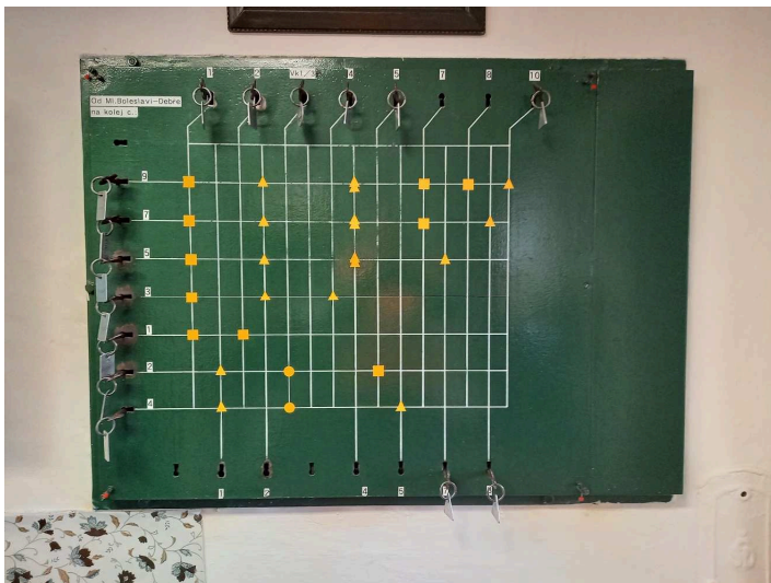
obrázek 247 – Ústřední zámek (potřebné tvary štítků od zámků výhybek a výkolejek vyznačeny na průsečících)
