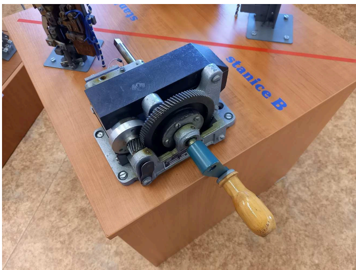
obrázek 299 – Hradlový induktor (demontovaný)
