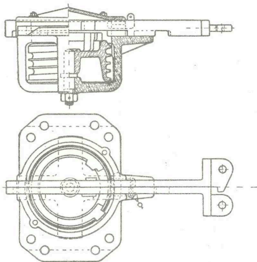
obrázek A.7 – Mechanický závorník
