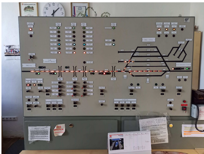
obrázek 29 – Příklad indikační desky (novější typ)
