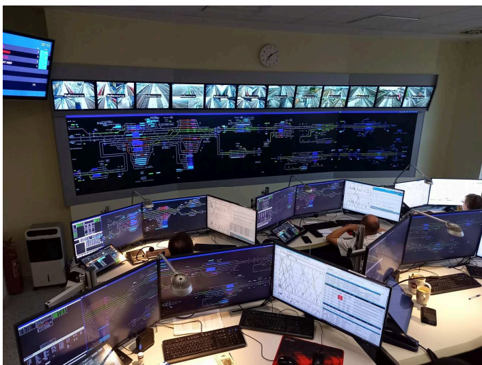
obrázek 369 – Pracoviště dálkového ovládání ZZ (centrální dispečerské pracoviště)
