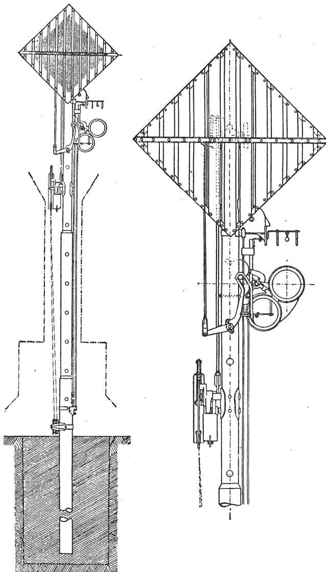
obrázek A.17 – Seřadovací mechanické návěstidlo
