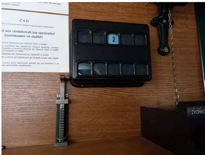
obrázek 252 – Kolejový číselník klíčového (bubnového) přístroje
