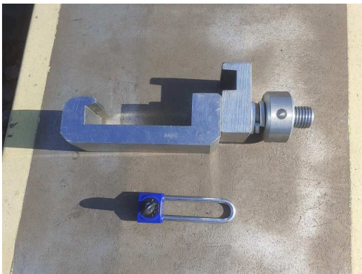
obrázek 125 – Přenosný zámek PHS malý (starší typ)
