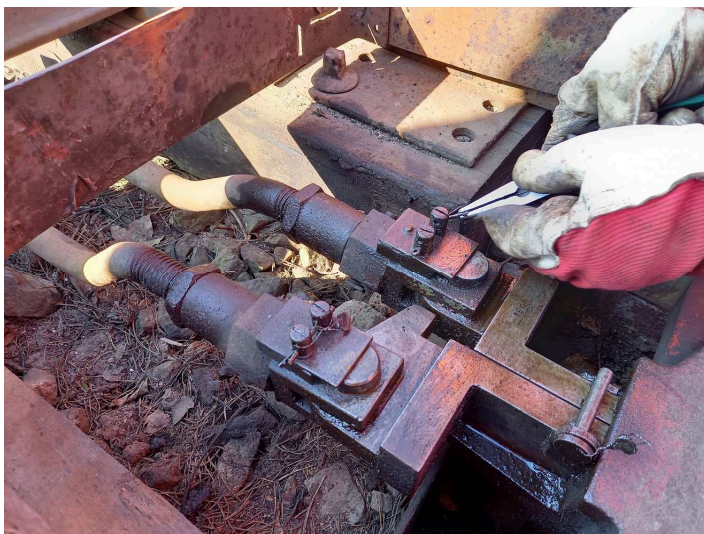
obrázek 187 – Sejmutí plomby na drátu
