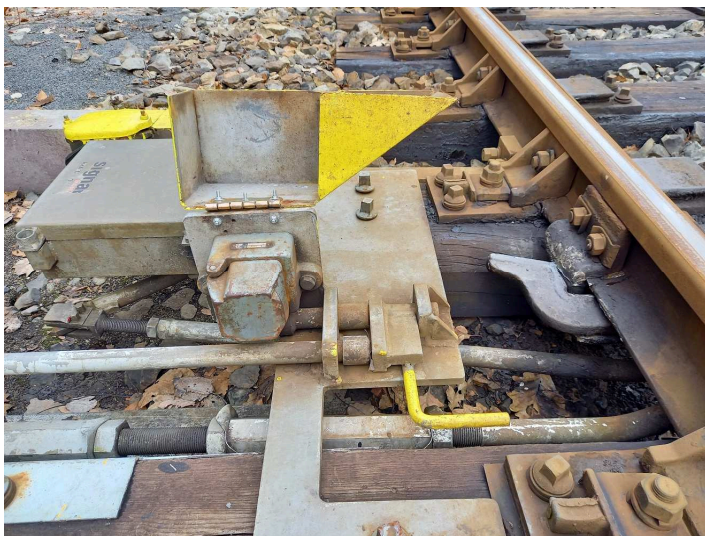
obrázek 110 – Spojovací zámek výrobce AK signal Brno (součást samovratného přestavníku)
