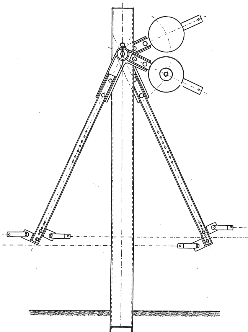
obrázek A.15 – Pákový dotahovač
