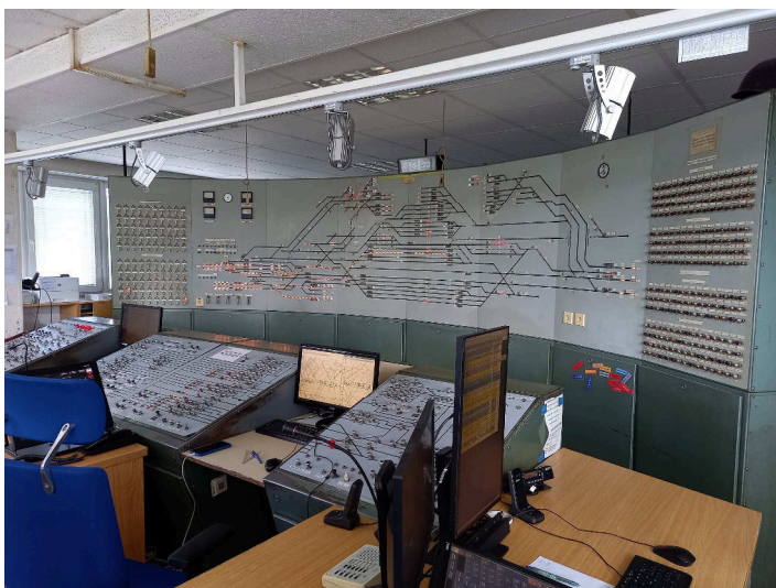
obrázek 341 – Ovládací stůl a indikační deska RZZ cestového systému se skupinově přestavovanými výhybkami (výkolejkami)
