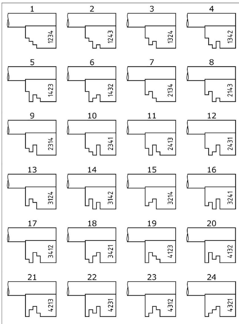
obrázek A.44 – Typy klíčů mechanických zámků
