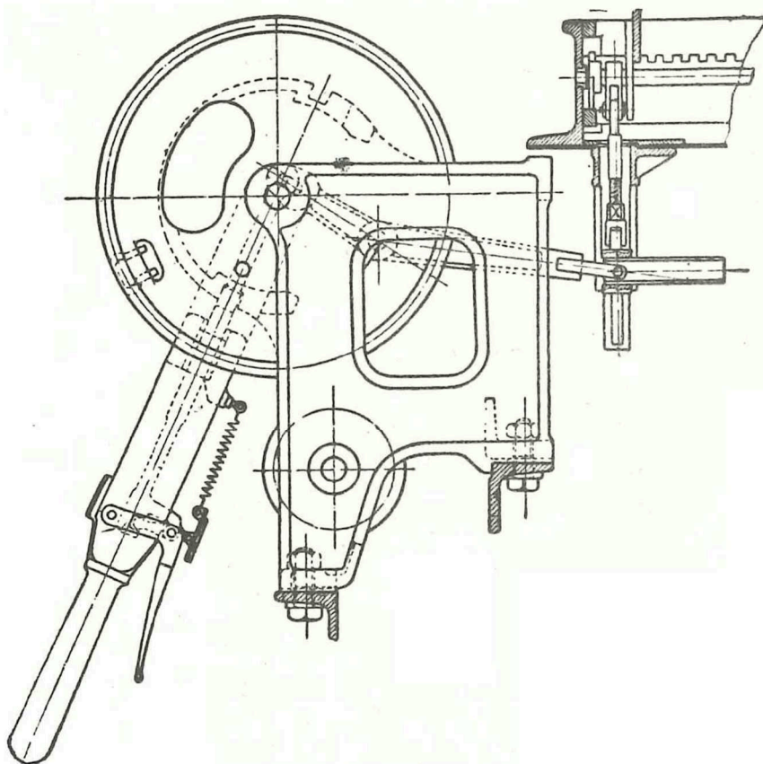
obrázek A.24 – Dvoupolohová páka
