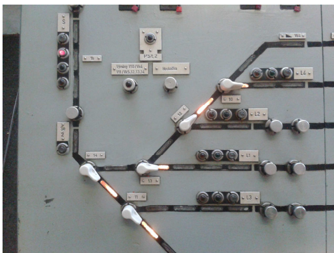
obrázek 337 – Detail kolejového reliéfu s indikačními a ovládacími prvky
