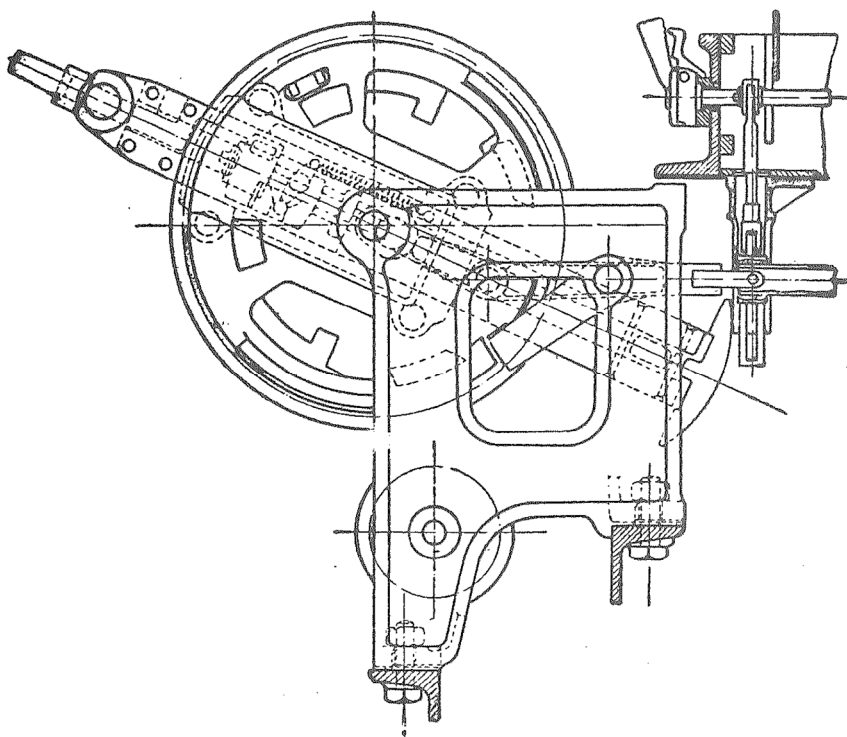
obrázek A.25 – Třípolohová páka
