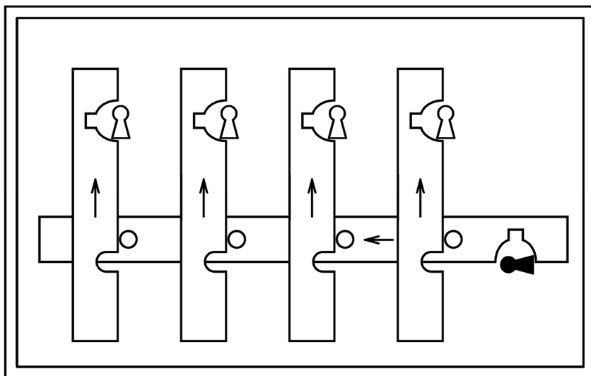
obrázek A.32 – Ústřední zámek s vyznačením závislostí
