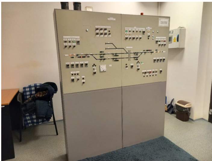
obrázek 340 – Indikační deska RZZ cestového systému se skupinově přestavovanými výhybkami (výkolejkami)
