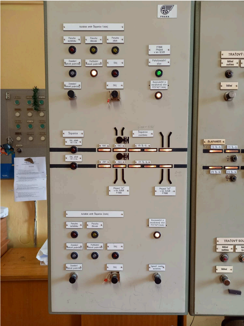
obrázek 392 – Příklad ovládacích a indikačních prvků automatického bloku ABE-1 na indikační desce
