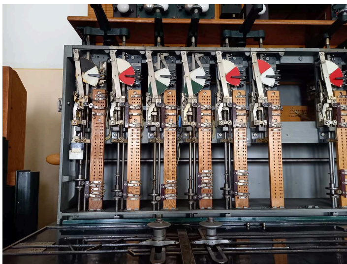
obrázek 295 – Hradlové závěry v hradlové skříni (sejmutý kryt hradlové skříně)
