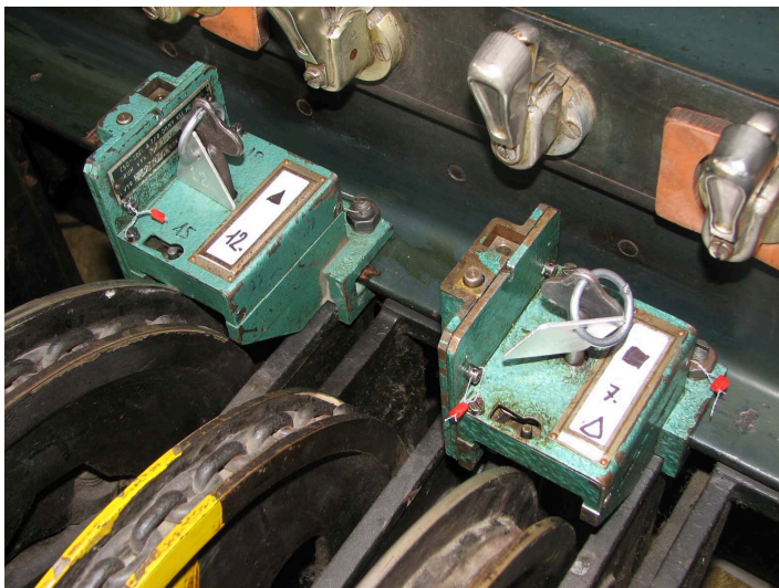
obrázek 277 – Pákový zámek (u jednoduché páky)
