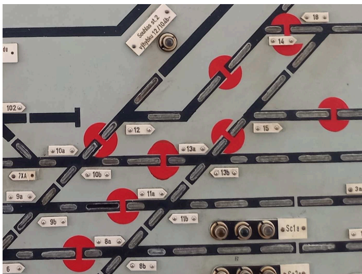
obrázek 230 – Grafické provedení neprofilového styku na indikační desce
