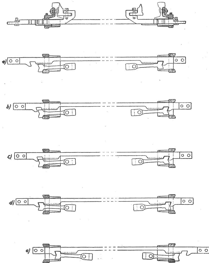
obrázek A.12 – Chod rybinového závěru výhybky s vyznačením změn fází v provedení s postupným chodem jazyků
