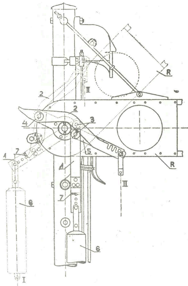
obrázek A.14 – Činnost rozvěšovacího zařízení jednoramenného mechanického návěstidla
