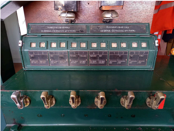
obrázek 285 – Kolejové číselníky a kolejové závěrníky
