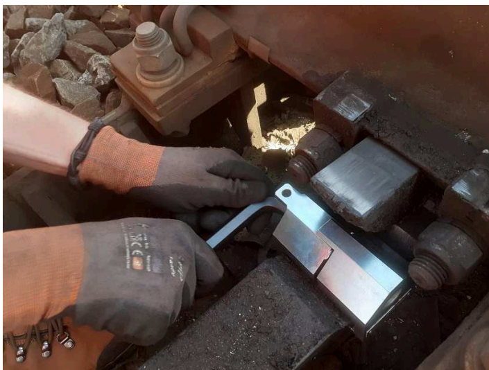
obrázek 145 – Dotažení PZČZ pomocí INBUS klíče
