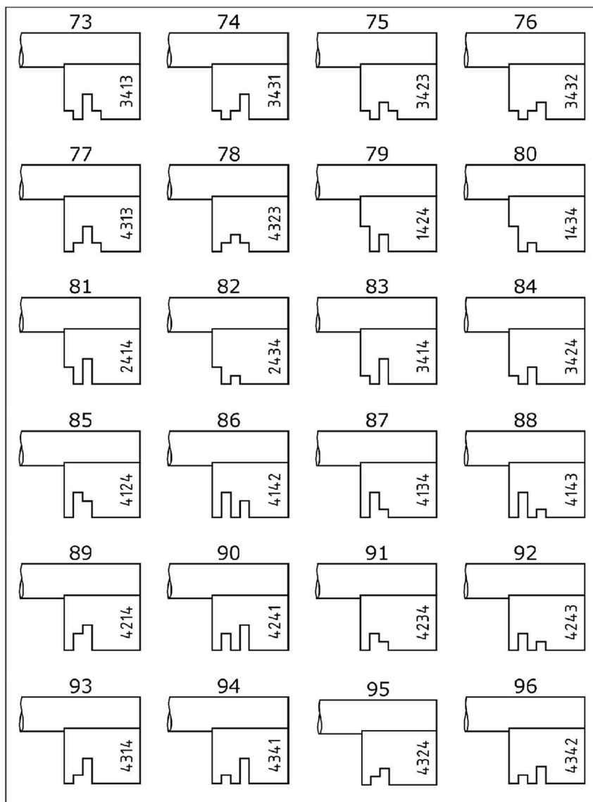
obrázek A.44 – Typy klíčů mechanických zámků (dokončení)
