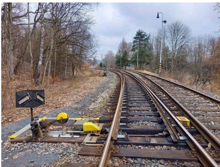
obrázek 57 – Výhybka se samovratným přestavníkem
