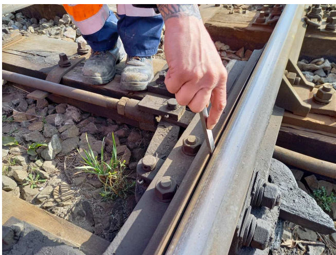
obrázek 84 – Západková zkouška – přestavení výhybky a přilehnutí jazyka k opornici (závěr jazyka se neuzavřel)
