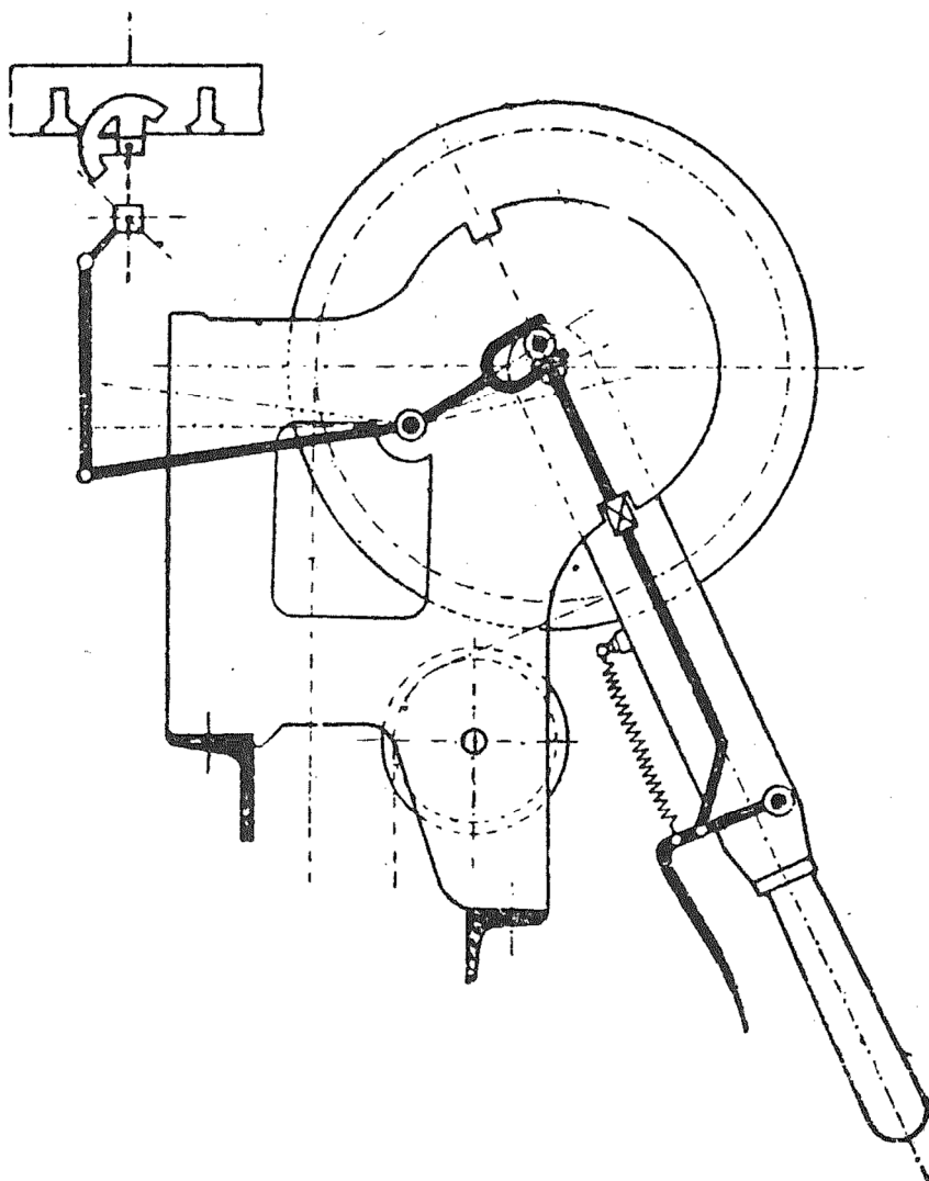
obrázek A.22 – Závislost páky na pravítkách
