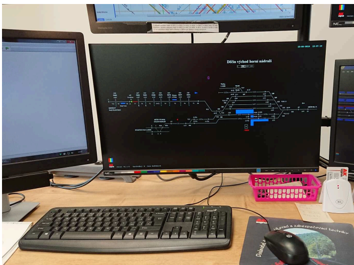
obrázek 376 – Jednotné obslužné pracoviště SZZ RZZ-DRS
