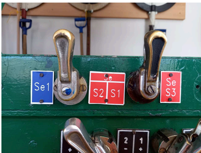
obrázek 267 – Označovací štítek klíčky pro rozsvícení návěsti „Posun dovolen“ světelného seřaďovacího návěstidla (vlevo) a světelného hlavního návěstidla (uprostřed, vpravo)
