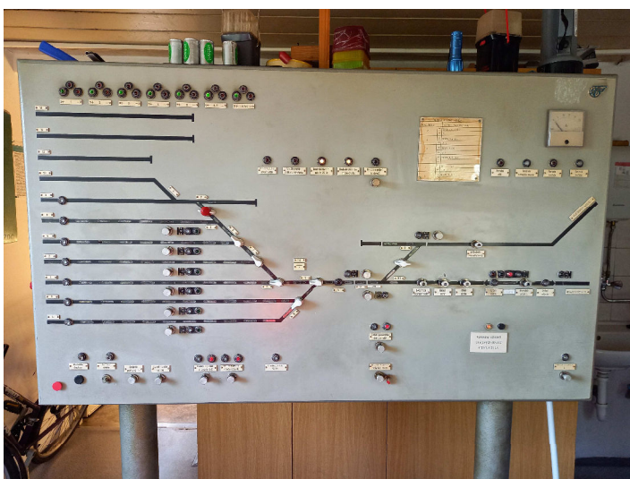
obrázek 363 – Závislé stavědlo SZZ TEST s řídícím stavědlem a závislými stavědly
