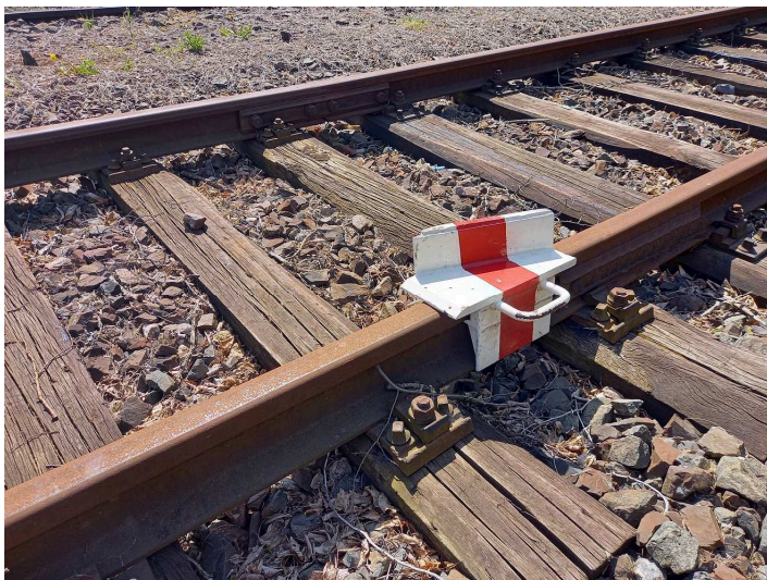
obrázek 93 – Přenosná výkolejka namontovaná na kolejnici
