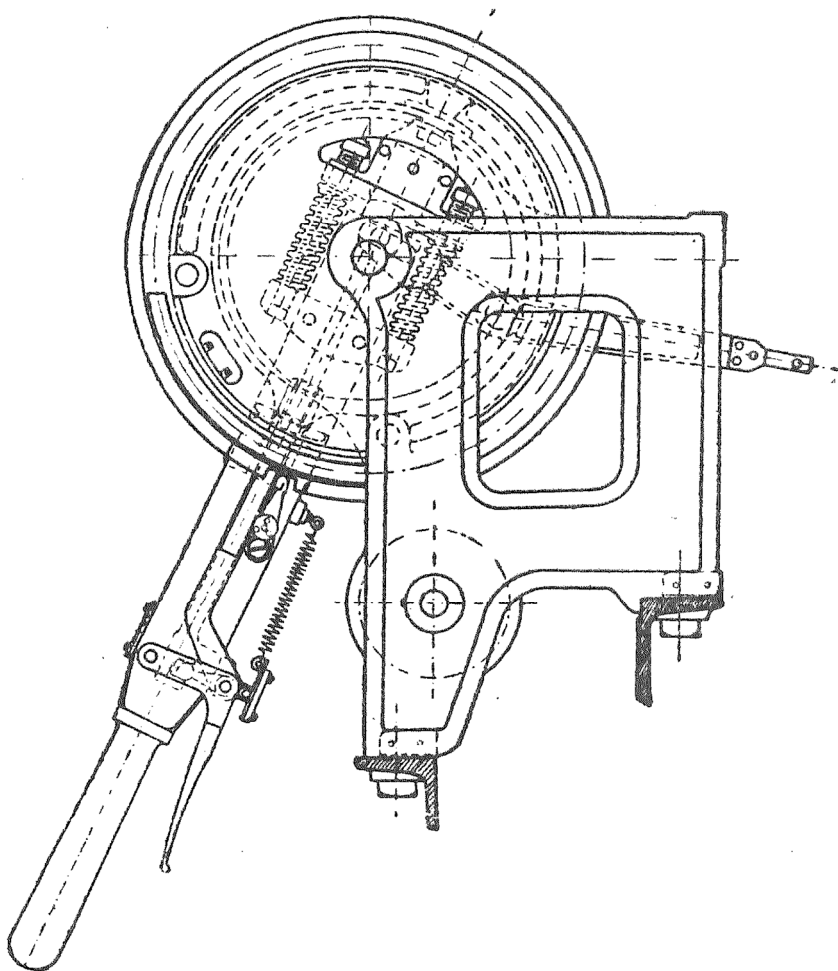
obrázek A.29 – Výměnová páka rozříznutelná
