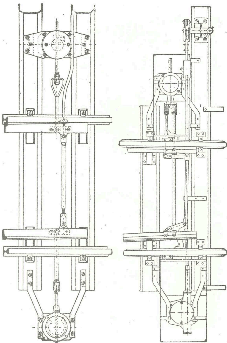
obrázek A.9 – Příklad umístění mechanického přestavníku a mechanického záporníku na výhybce
