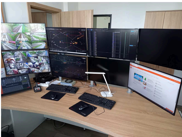
obrázek 373 – Jednotné obslužné pracoviště SZZ K-2002 pro dálkové ovládání ZZ
