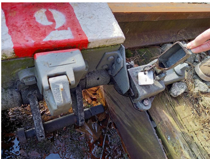
obrázek 115 – Výkolejka s dvěma jednoduchými výkolejkovými zámky, klíč od výměnového zámku lze vyjmout až po sklopení svodného klínu a uzamknutí svodného klínu ve sklopené poloze
