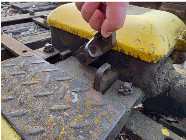
obrázek 151 – Elektrický výměnový zámek, po otočení závorovací páčky lze výhybku ručně přestavovat
