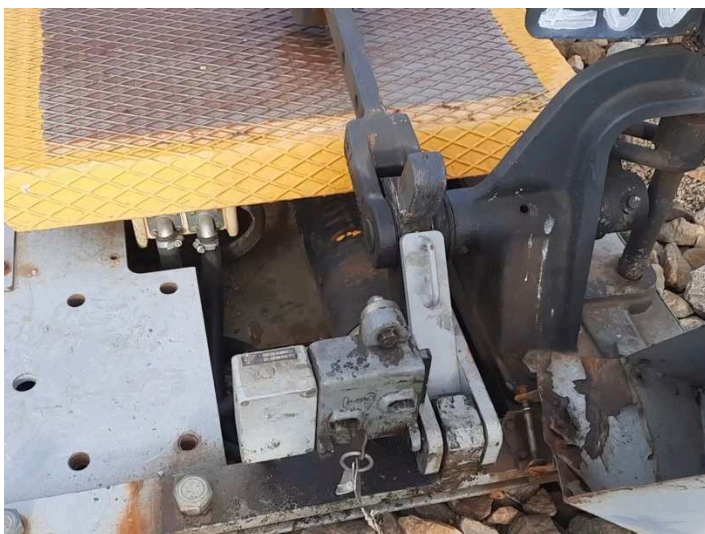
obrázek 111 – Spojovací zámek výrobce AŽD Praha (součást samovratného přestavníku)
