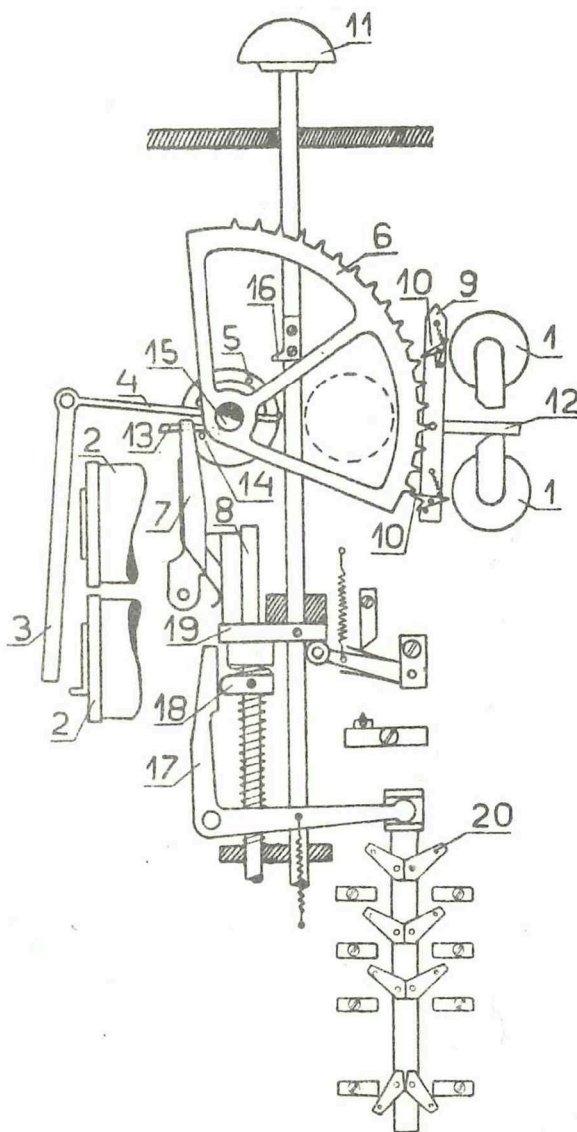
obrázek A.37 – Hradlový závěr na střídavý i stejnosměrný proud
