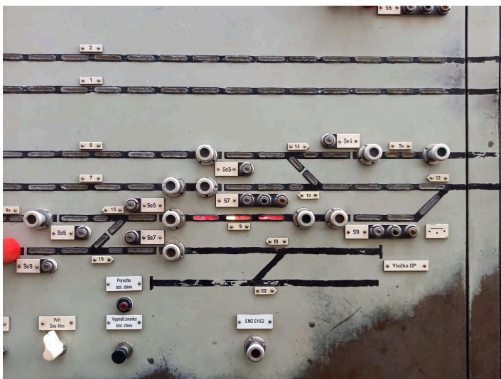
obrázek 339 – Detail kolejového reliéfu s indikačními a ovládacími prvky
