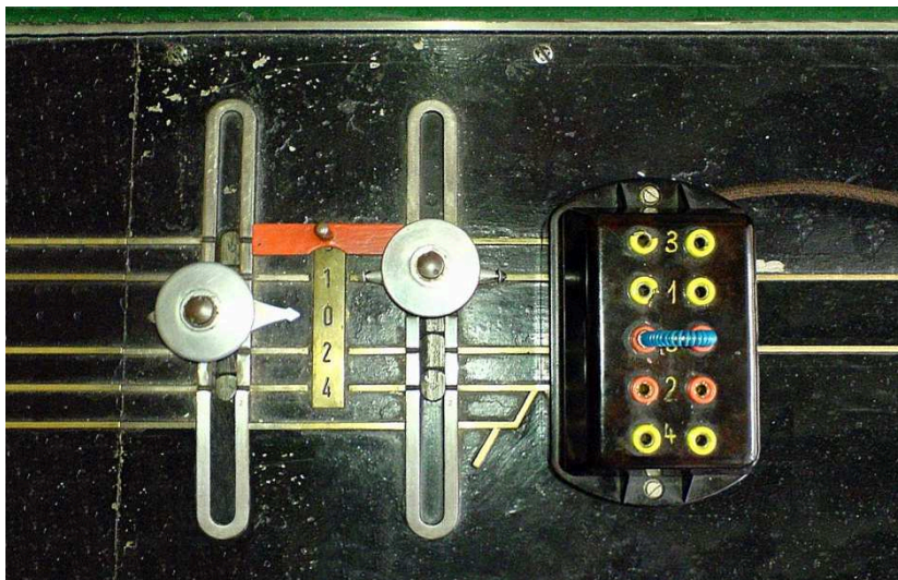
obrázek 313 – Kolíčkový zapojovač (horizontální provedení)
